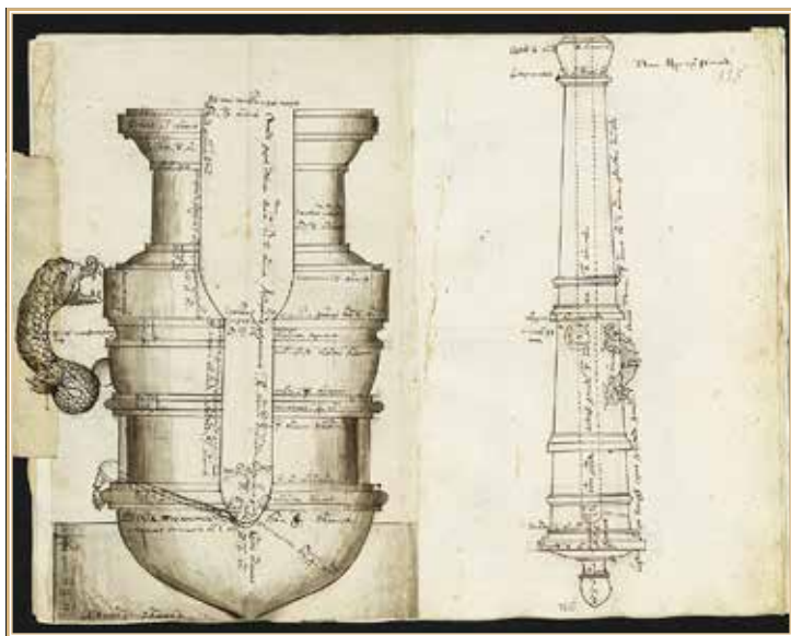
Чертеж мортиры и пушки.
