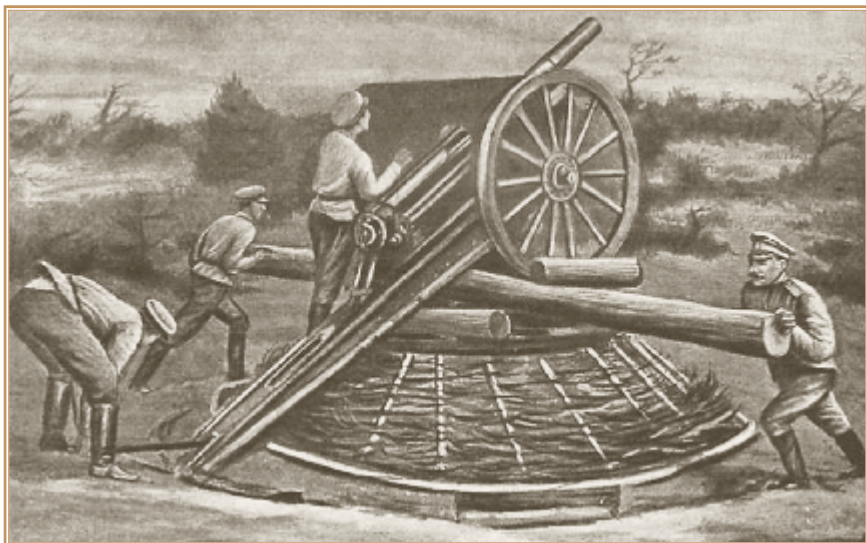
Полевое орудие на импровизированном зенитном станке из бревен
