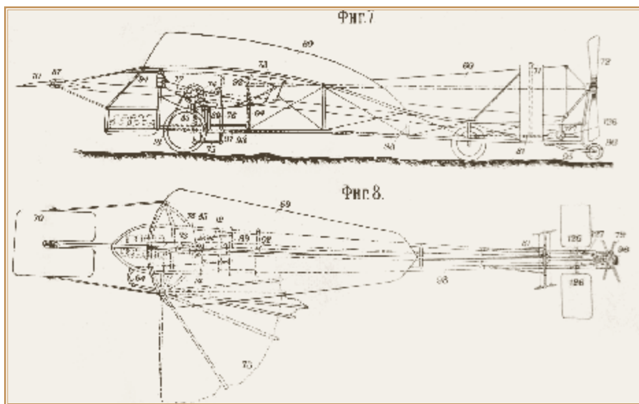
Чертеж аэроплана конструкции полковника С. Люпова
